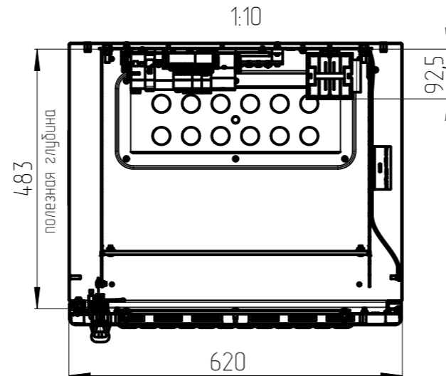
Вид сверху (закрытая дверь)
