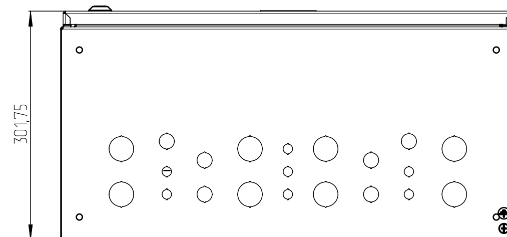
Вид снизу
