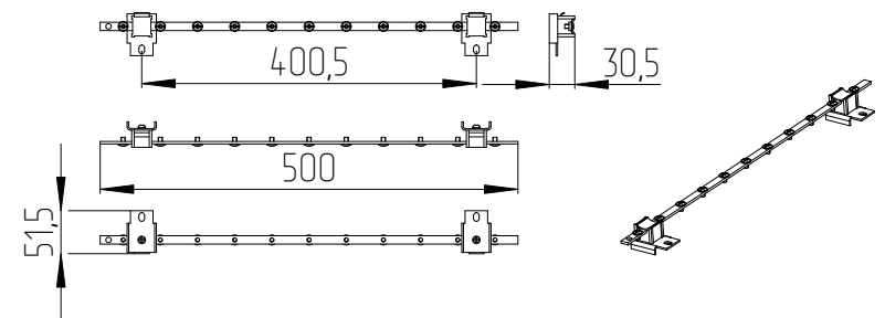
Панель заземления ПЗ-500.80А (ПЗ-500.200А)
